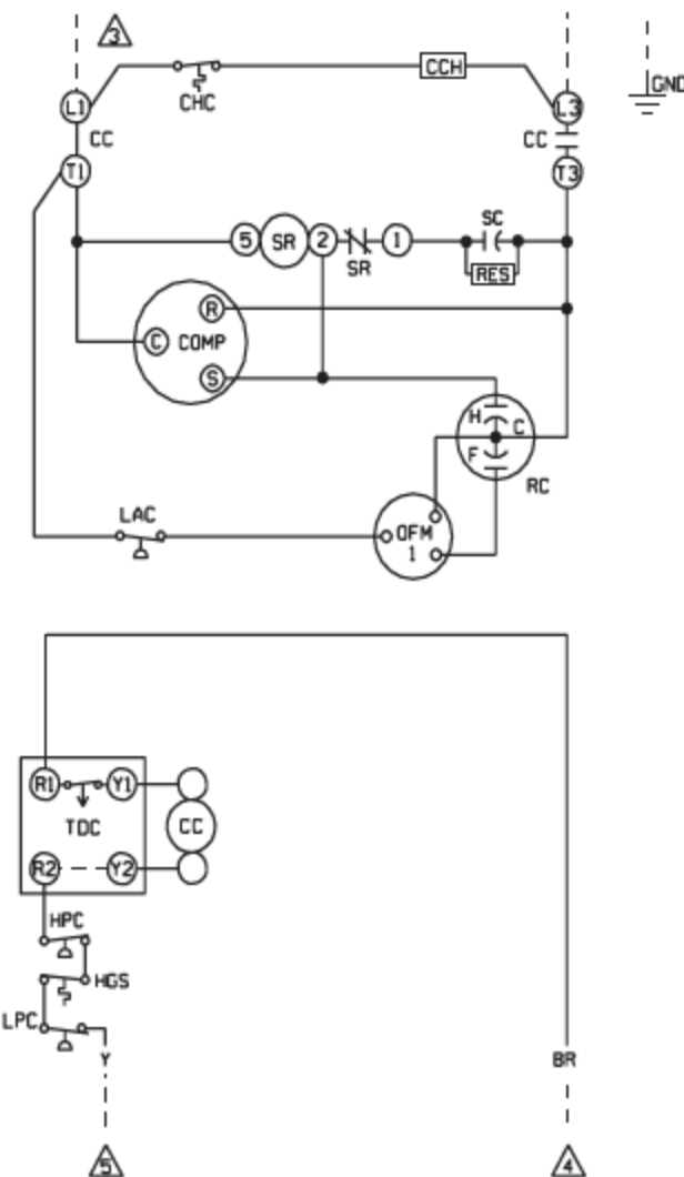
WIRING SCHEMATIC
